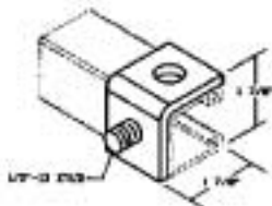
L14 1 Stud - 1 Hole Angle
